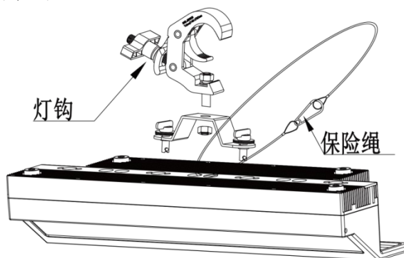
吊挂放置图
